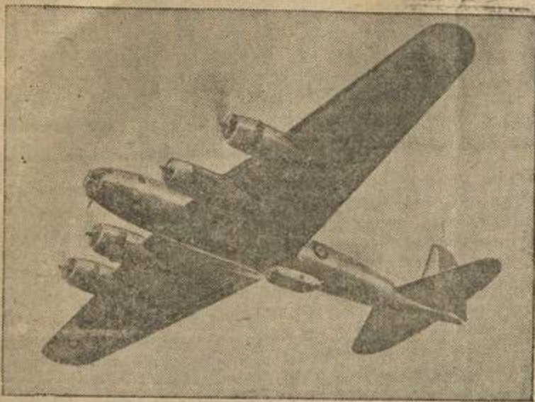
Американский бомбардировщик «Летающая крепость» на службе в английских воздушных силах. Скорость бомбардировщика превышает 300 миль в час, дальность полета 3500 миль, потолок 36000 футов, размах крыльев 105 футов, длина 70 футов, высота 15 футов. Бомбовый груз составляет несколько тонн.
