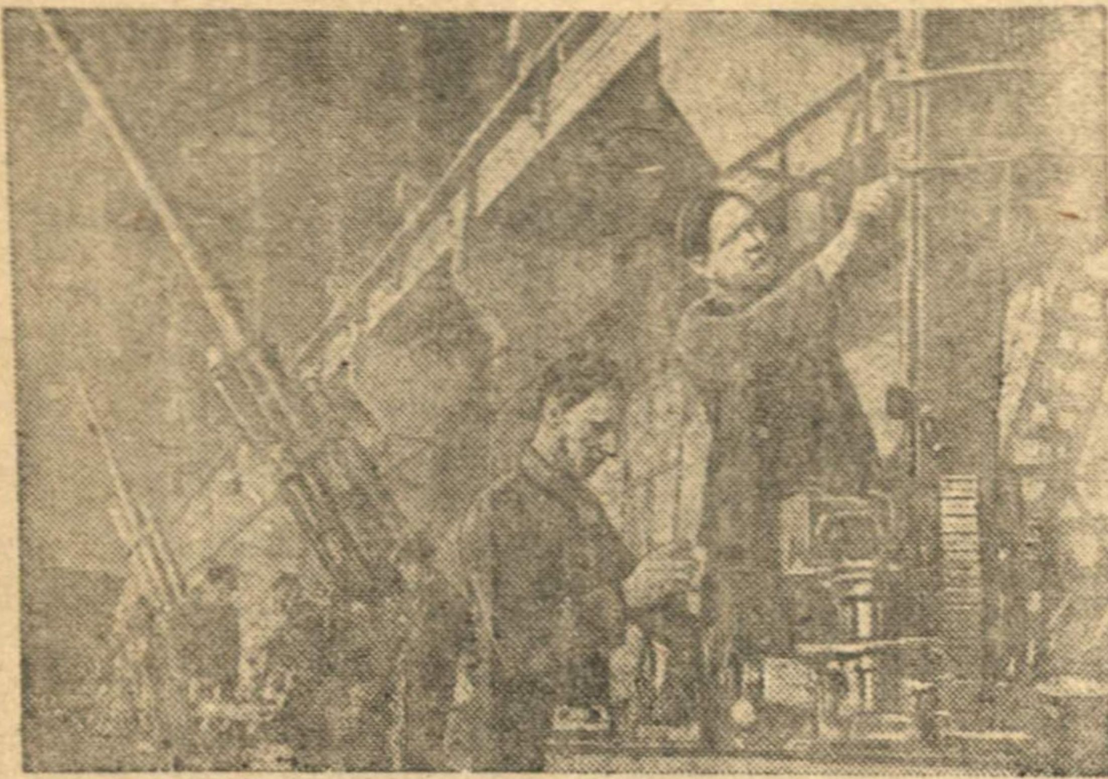
Н-ский артиллерийский завод. Сборка зенитных орудий. На переднем плане слесари-сборщики стахановцы Б. А. Сибирков (слева) и комсомолец К. В. Кондриков.
